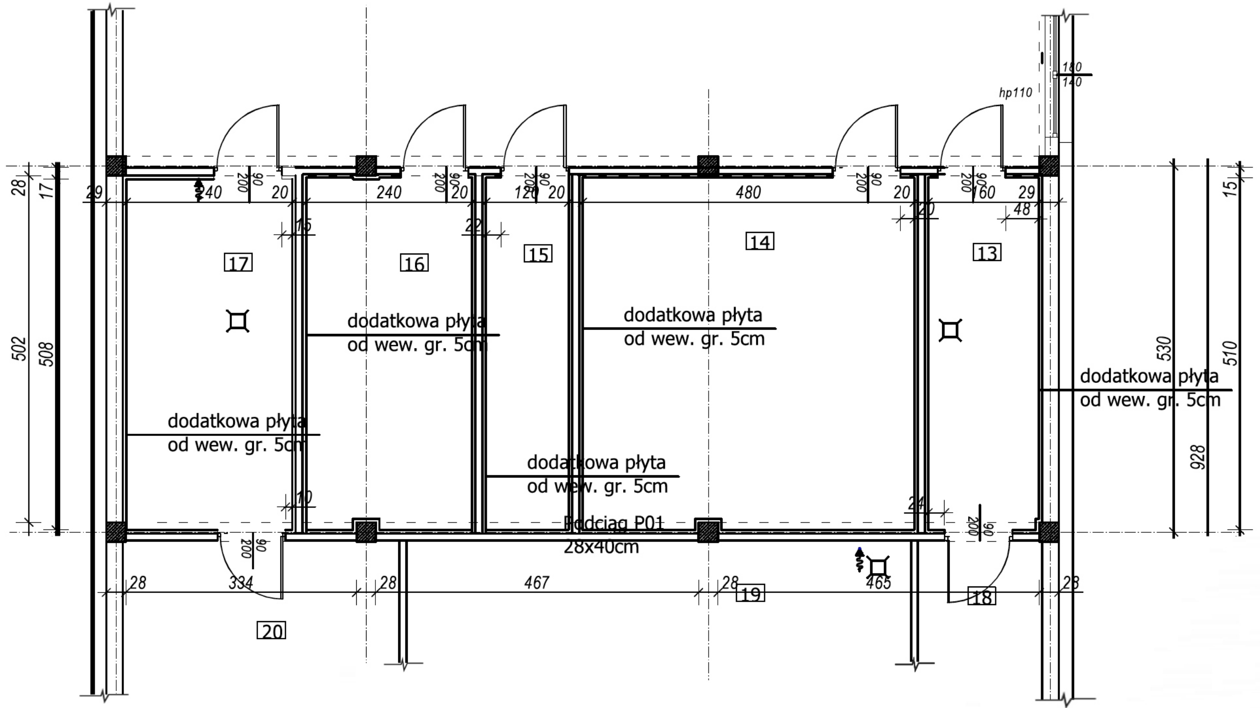
Załącznik nr. 1. Rzut z góry systemu komór procesowych.
